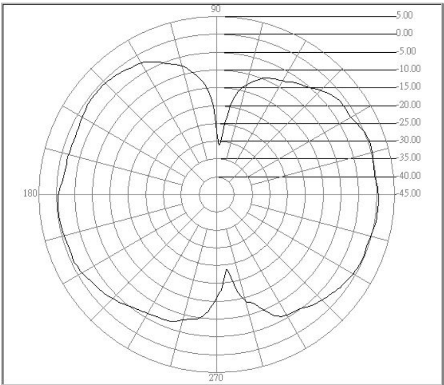
E-Plane
