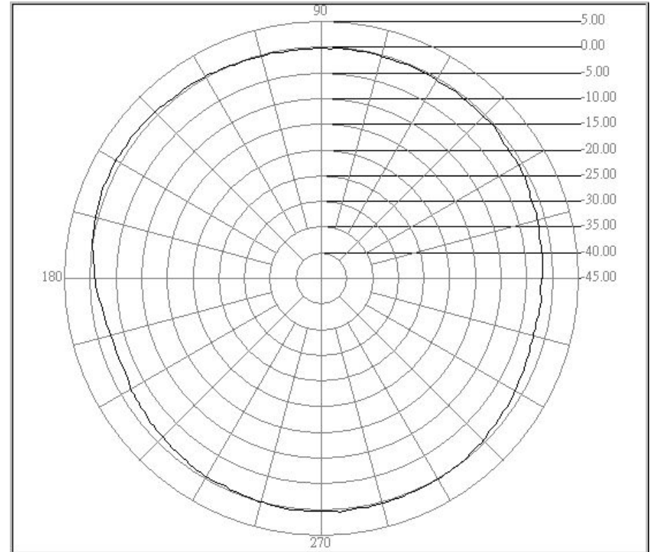
H-Plane
