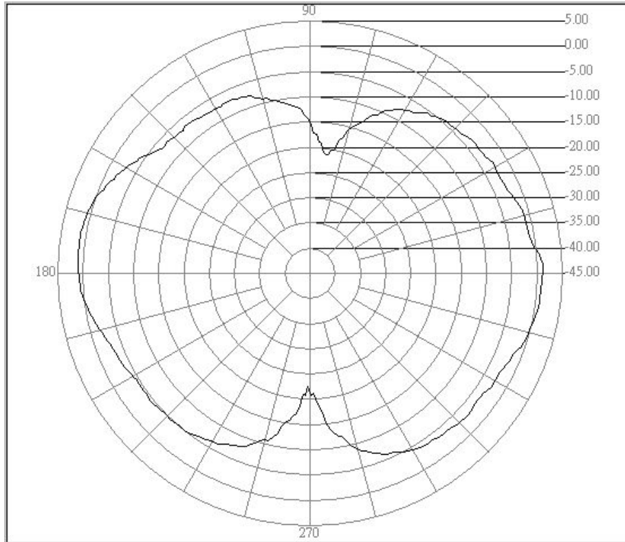
E-Plane
