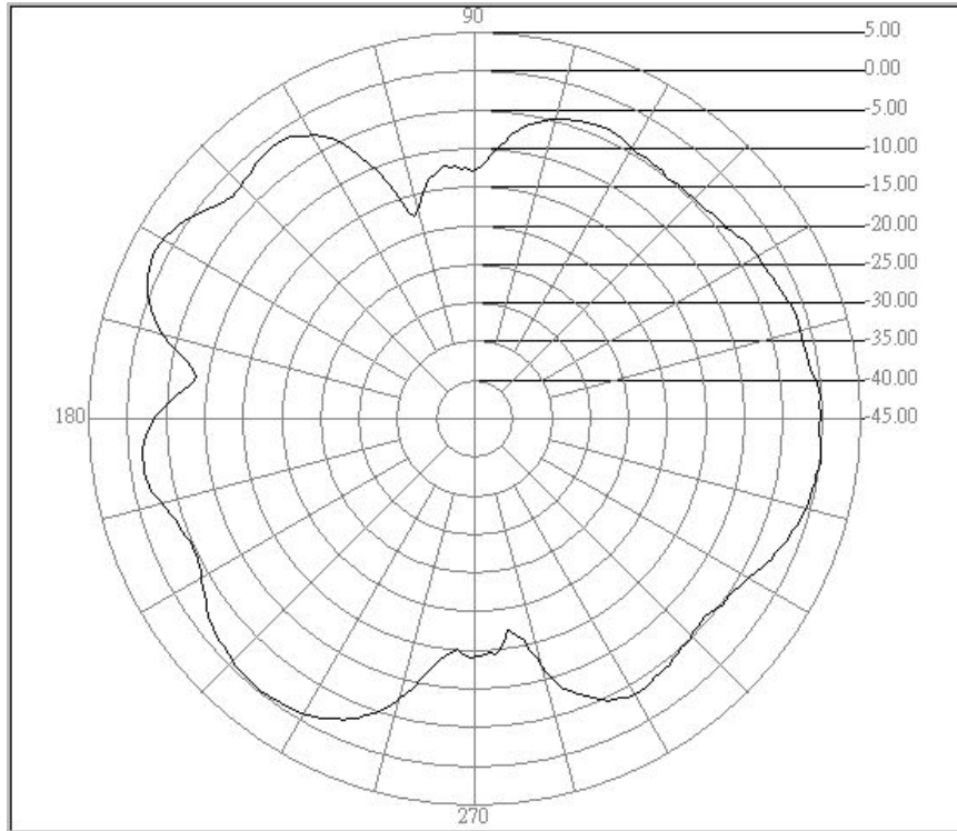
E-Plane
