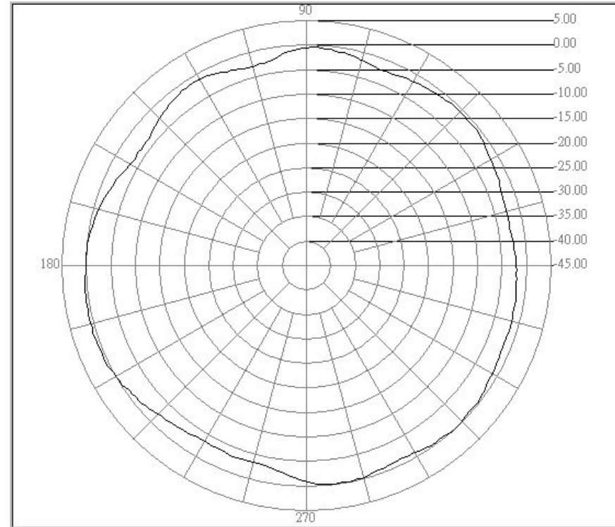
H-Plane
