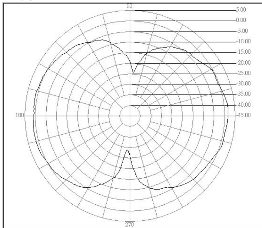
E-Plane
