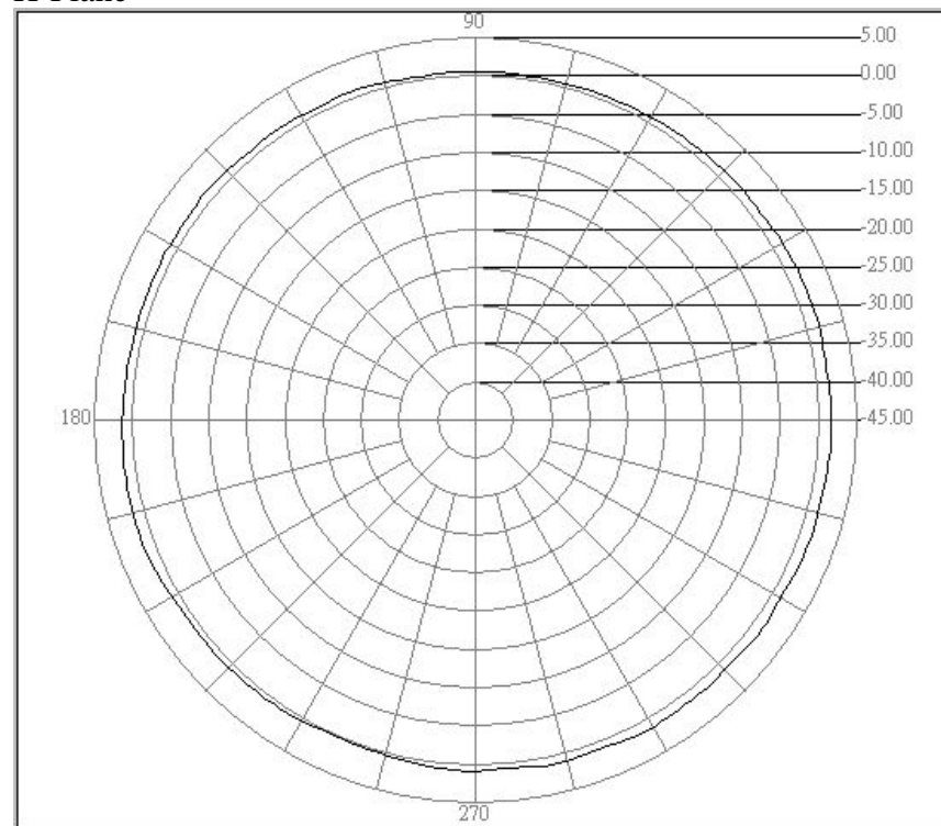
H-Plane
